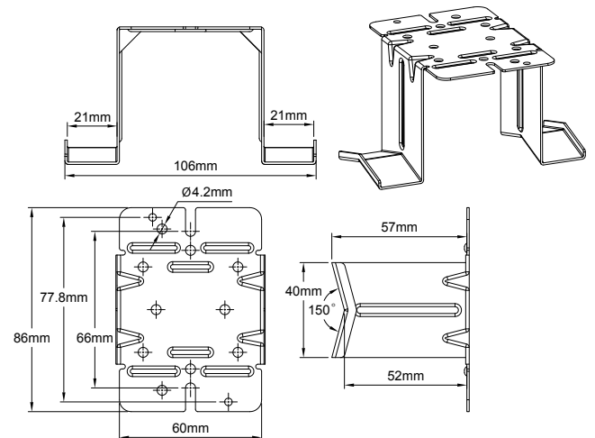
Тип 6УТРТВ499
